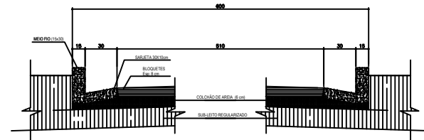
SECÇÃO ESQUEMÁTICA 3/ESCALA
