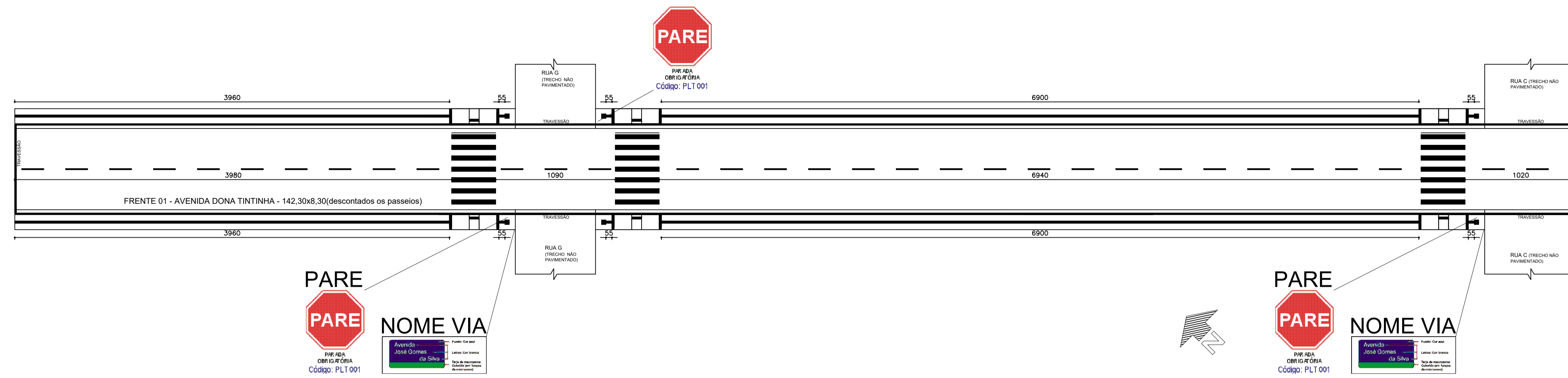
LAYOUT PLACAS-ACESSIBILIDADE 1:250
